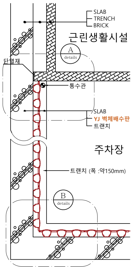
확대 평면도
