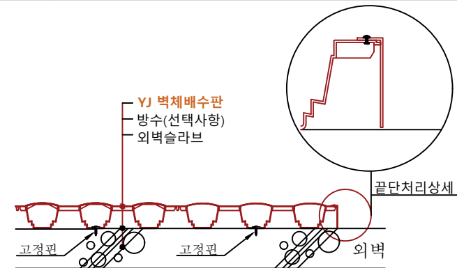
벽면/기둥과 만나는 부분 단면상세(몰딩사용)
