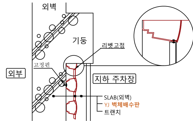
벽면/기둥과 만나는 부분 단면상세(몰딩사용)
