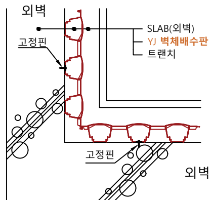
벽면 코너 부분 단면상세(표준)
