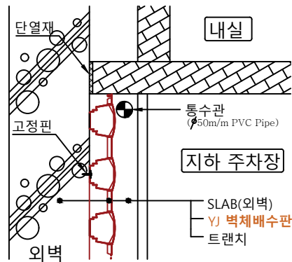
벽면/기둥과 만나는 부분 단면상세(표준)
